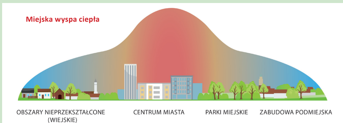
Rozkład temperatury w zależności od charakteru zabudowy
